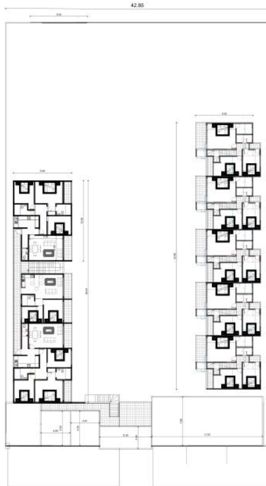
VUE EN PLAN R+1
